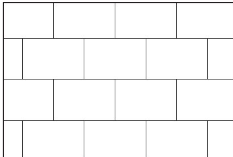
Motif de pose « lisière » 40 x 60
