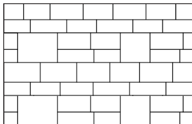
Module 1: 80 % Module 2: 20 % Motif de pose «lisière modulaire»
