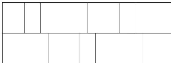
Motif de pose « lisière » 3 morceaux Superficie pi 2 ou m 2 couverte pour chaque dimension 20 x 40 : 16 % • 40 x 40 : 34 % • 40 x 60 : 50 %
