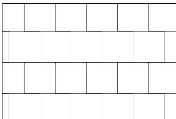
Motif de pose « lisière » 40 x 40
