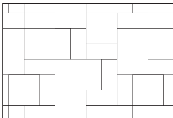
Motif de pose « modulaire » 3 morceaux Superficie pi 2 ou m 2 couverte pour chaque dimension 20 x 40 : 28 % • 40 x 40 : 28 % • 40 x 60 : 44 %
