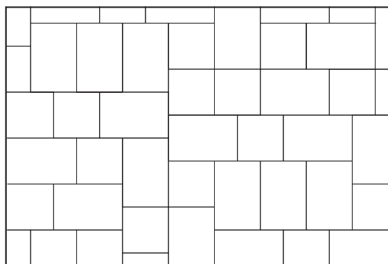
Motif de pose « modulaire » 2 morceaux Superficie pi 2 ou m 2 couverte pour chaque dimension 40 x 40 : 27 % • 40 x 60 : 73 %
