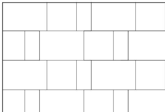
Motif de pose « lisière » 3 morceaux Superficie pi 2 ou m 2 couverte pour chaque dimension 20 x 40 : 16 % • 40 x 40 : 30 % • 40 x 60 : 54 %
