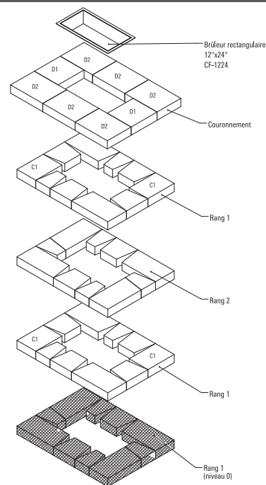
Vue explosée du foyer
