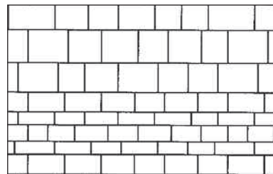
Combinaison des modules 1 et 2 en assemblage lisière
